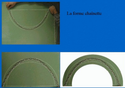
Les forces dans les voûtes
